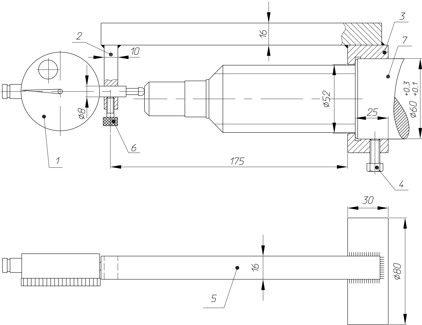
Рисунок 77 – Приспособление для замера осевого люфта первичного и вторичного валов
