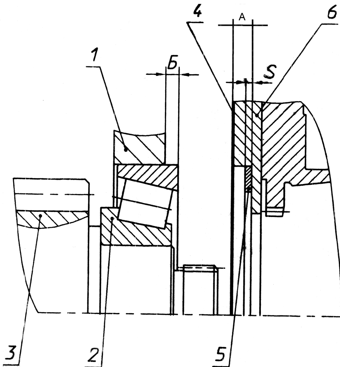
Рисунок 80 – Подбор установочных прокладок для обеспечения беззазорного торцового упора заднего подшипника промежуточного вала с проставкой демультипликатора
