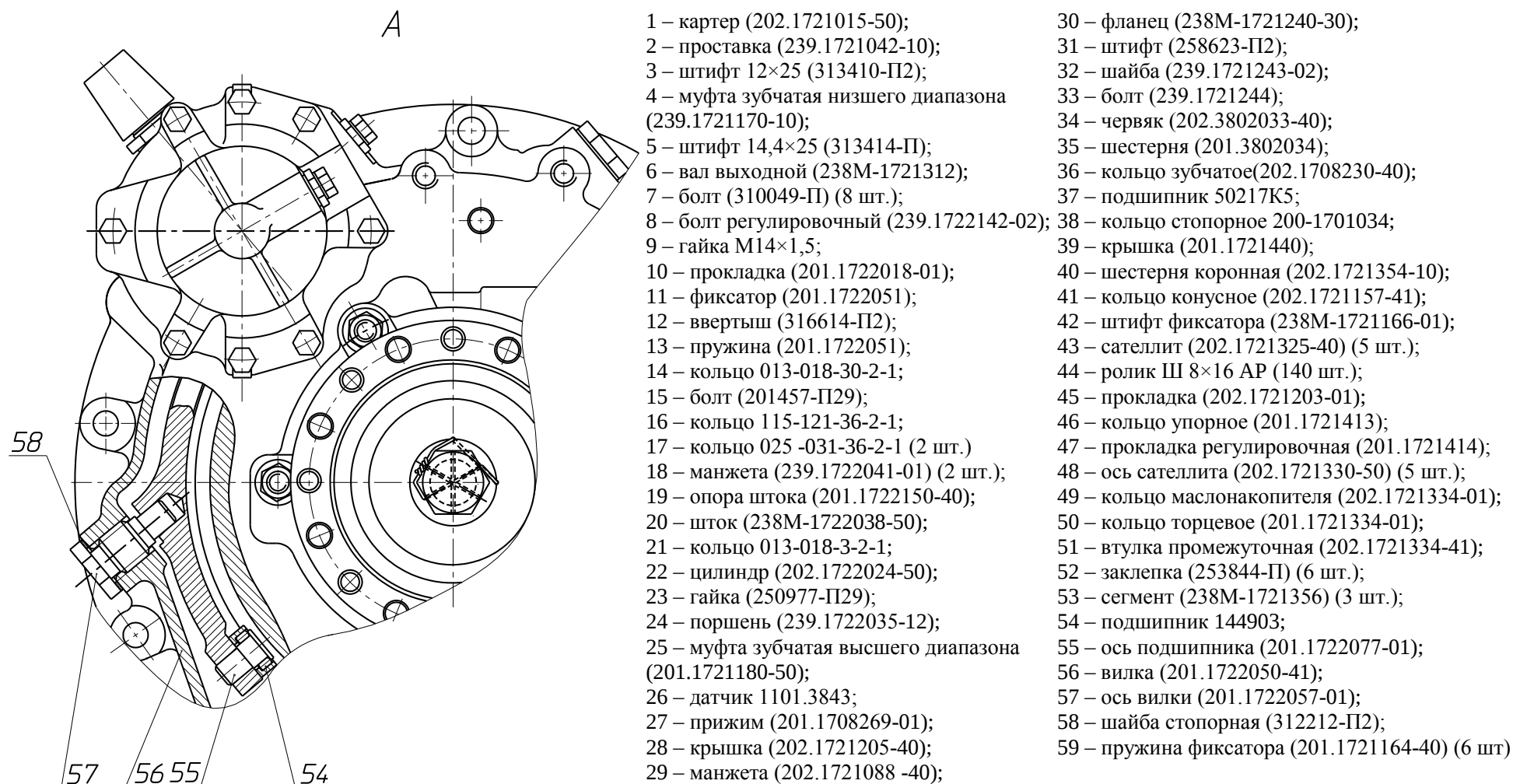
Рисунок 19 (продолжение) – Демультипликатор в сборе КП ЯМЗ-239
