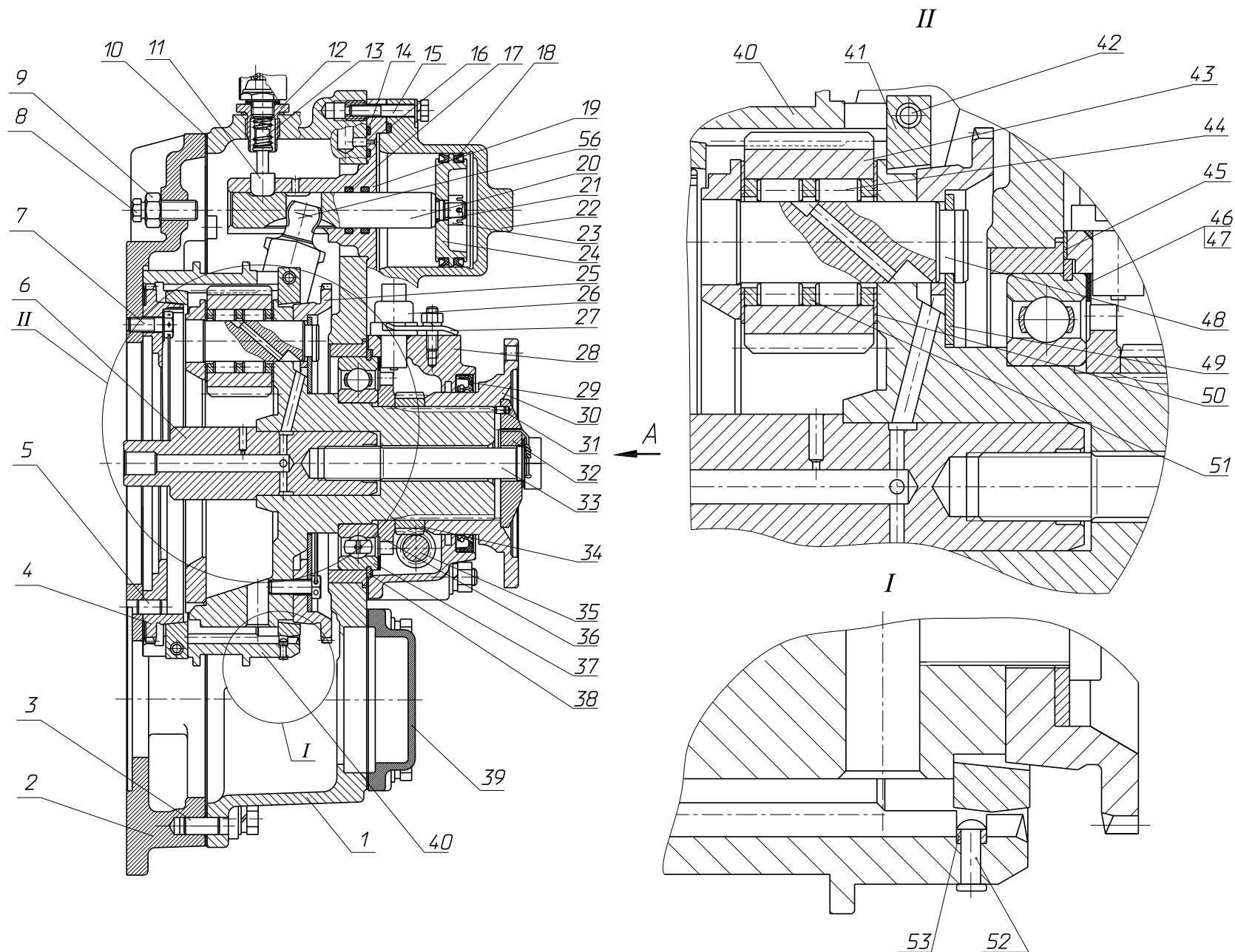
Рисунок 19 – Демультипликатор в сборе КП ЯМЗ-239
