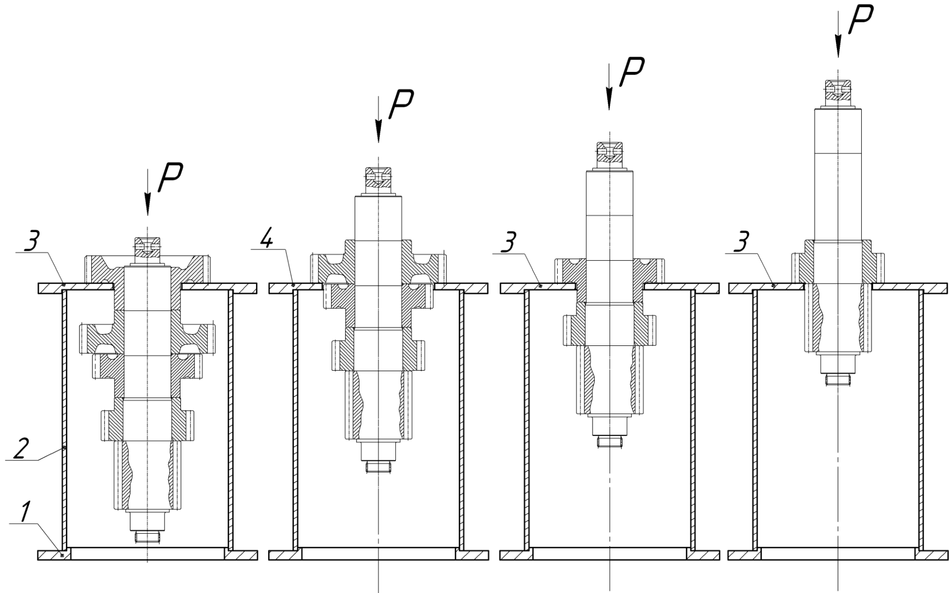
Рисунок 45 – Конструкция подставки и последовательность спресовки шестерён вала промежуточного КП типа ЯМЗ-239 1 – основание подставки; 2 – стойка; 3 – диск опорный Ø 100 мм; 4 – диск опорный Ø 180 мм (шестерни 5-ой передачи). Детали 1 и 2 соединяются между собой электродуговой сваркой.
