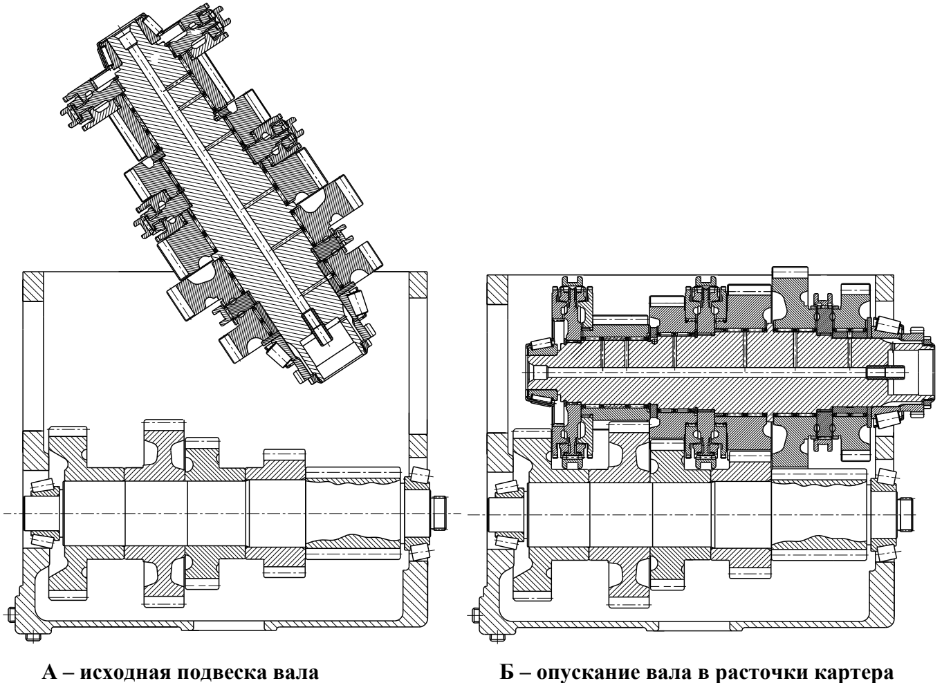
Рисунок 73 – Установка вторичного вала
