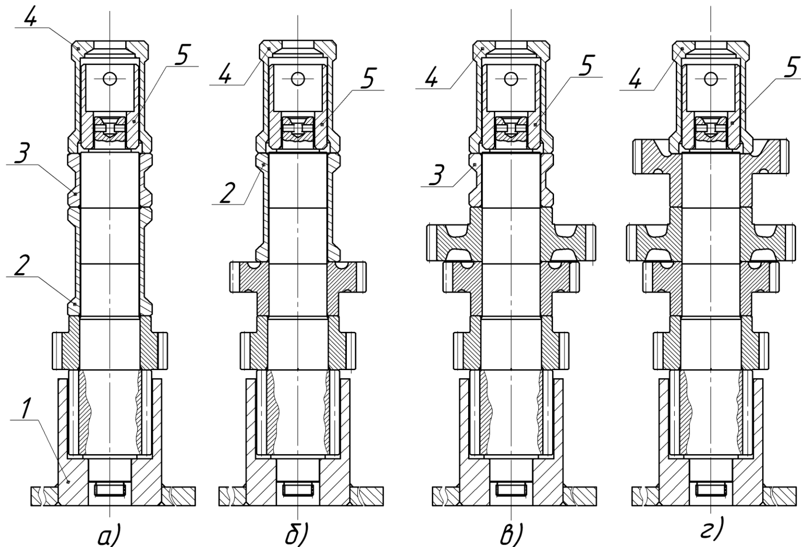
Рисунок 47 – Последовательность сборки вала промежуточного КП ЯМЗ-239 методом запрессовки:
