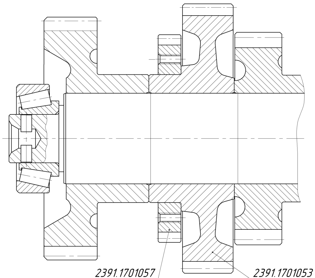
Рисунок 7 – Фрагмент вала промежуточного в сборе, дет. 2391.1701047, КП ЯМЗ-2391 (остальное аналогично приведенному на рисунке 5)
