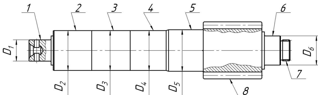
Рисунок 63 – Вал промежуточный
